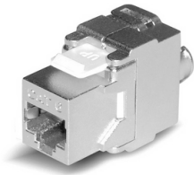
Module KS-T 5 1/8 toolless Cat.5e afgeschermd
